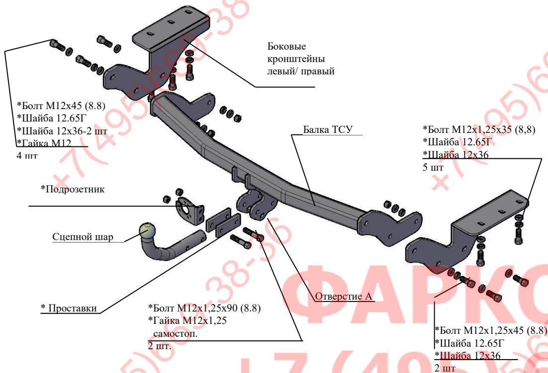
Рис.1 Тягово-сцепное устройство 7833.
